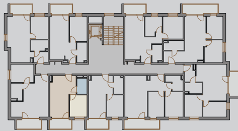
RZUT KONDYGNACJI
